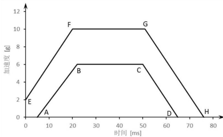
图 4 侧面碰撞自动触发加速度通道
