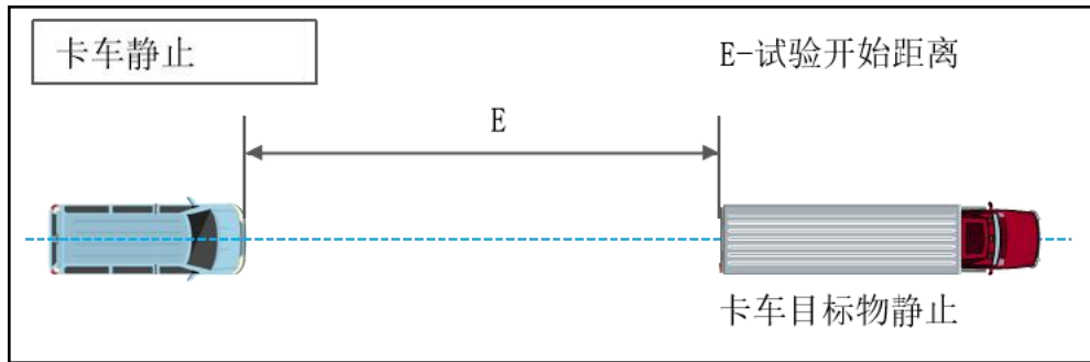
图 10 FCW 卡车静止工况（续）
