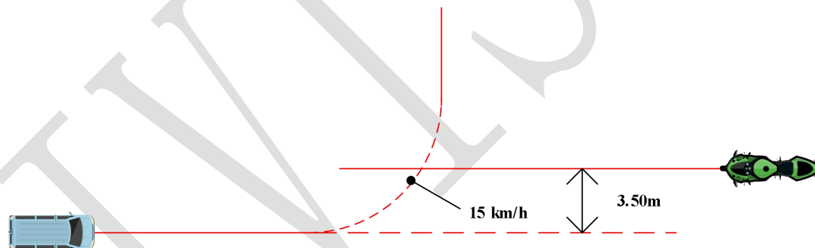
图 16 主车左转踏板摩托车直行工况
