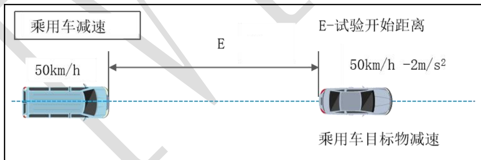
图 15 AEB 乘用车减速工况
