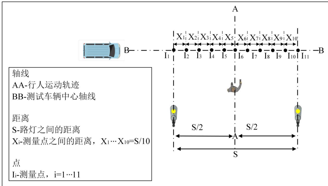
图 7 主车路径上的照度测量
