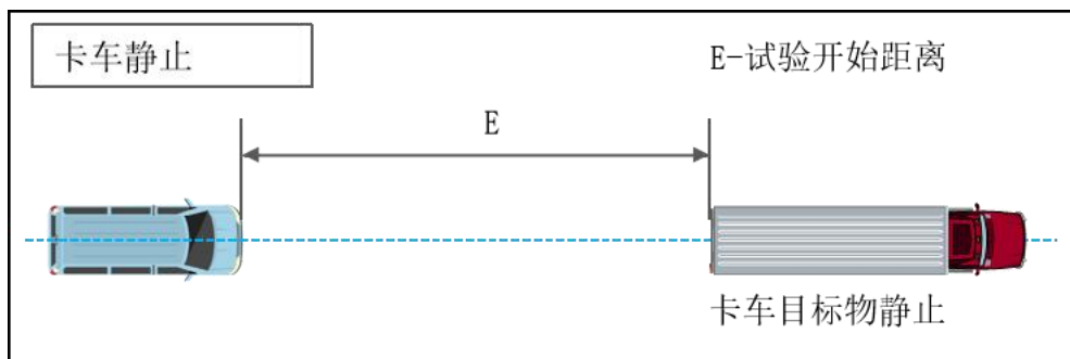
图 12 卡车静止工况
