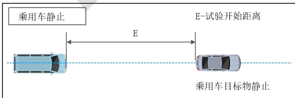
图 10 FCW 乘用车静止工况
