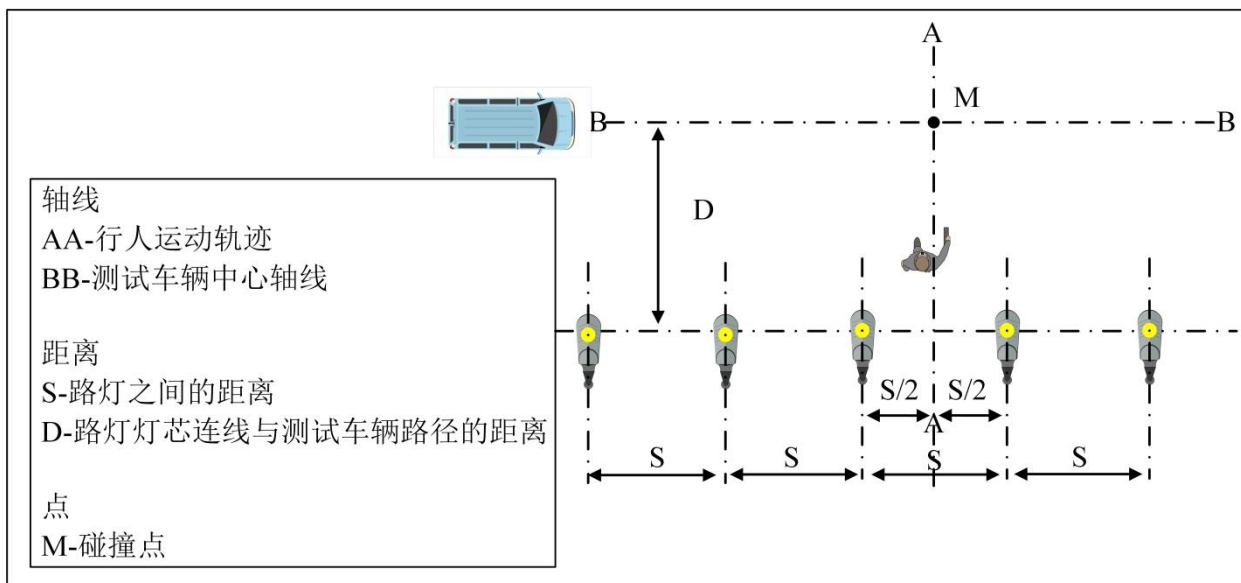
图 9 路灯安装位置
