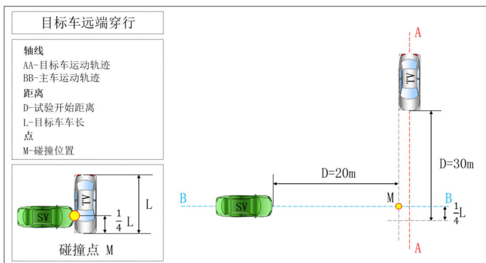
图 A. 3 目标车远端穿行工况
