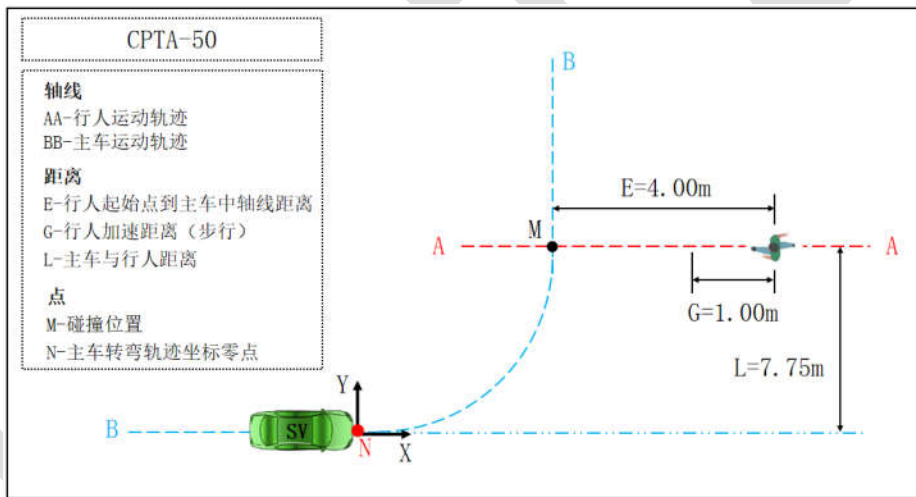
图 B. 4 CPTA-50 工况
