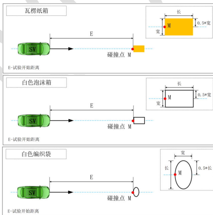
图 C.1 异形目标物静止工况
