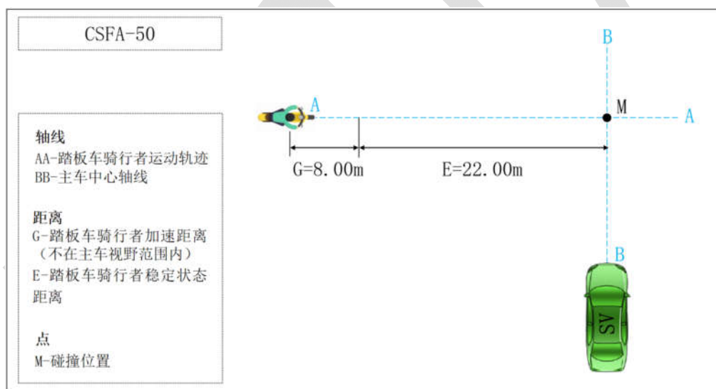
图 B.8 CSFA-50 工况
