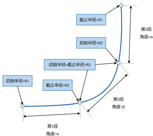
图 B. 10 主车左转路径要求
