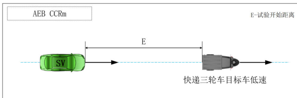
图 A. 7 三轮车目标车低速工况
