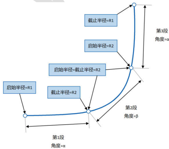
图 B. 5 主车左转路径要求
