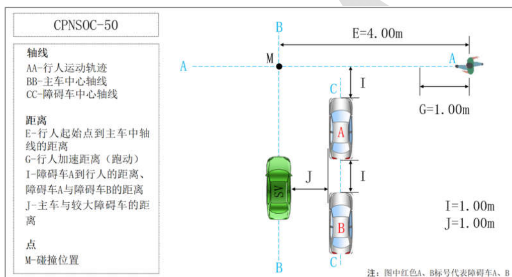
图 B.3 CPNSOC-50 工况
