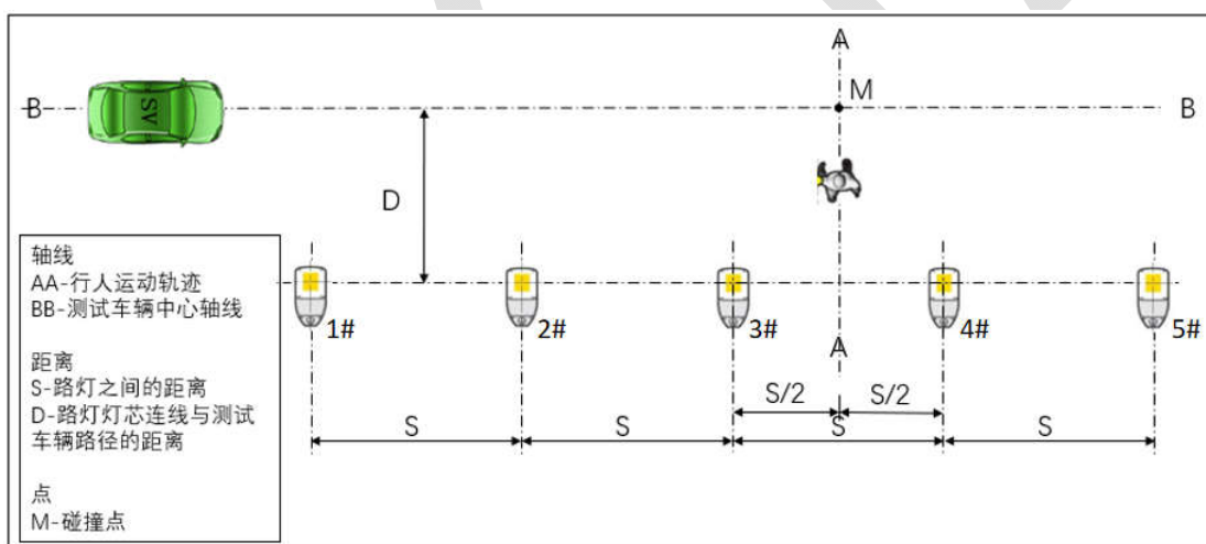
图 B.14 路灯安装位置
