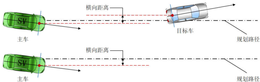
图1 横向距离示意图
