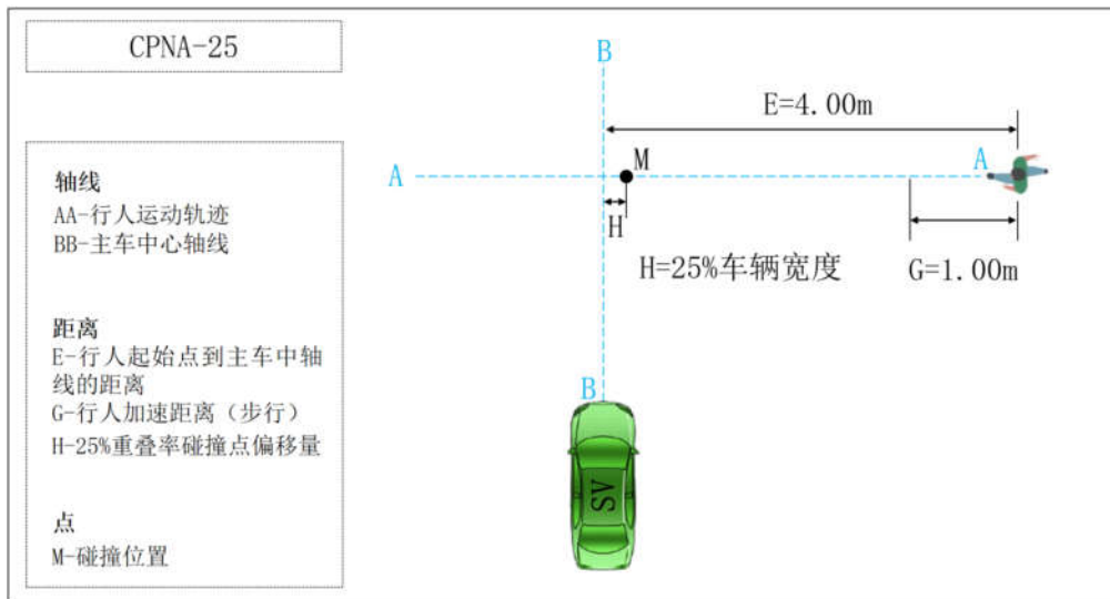
图 B. 2 CPNA-25 工况
