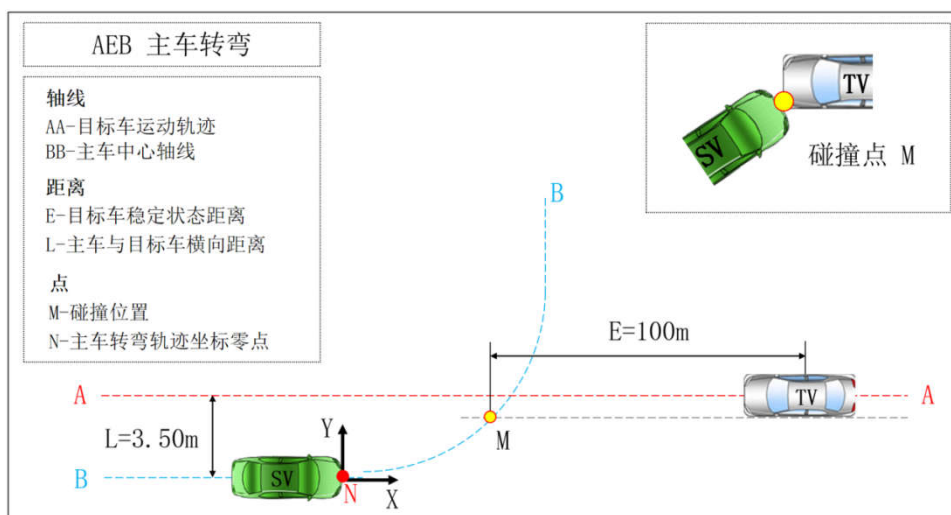
图 A. 4 主车左转-目标车对向直行工况
