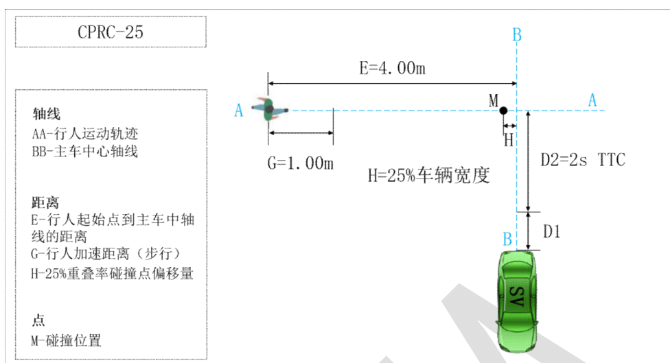
图 B. 6 CPRC-25 工况
