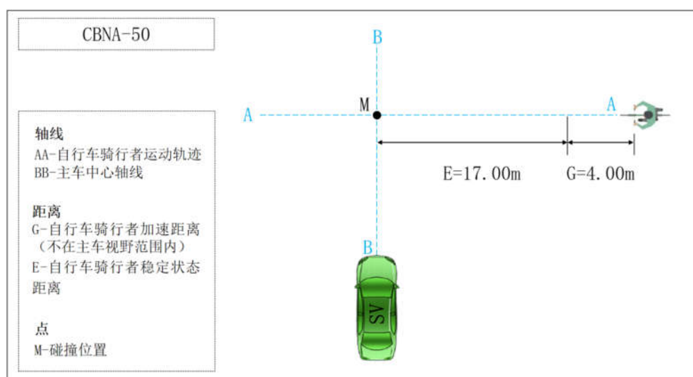
图 B.7 CBNA-50 工况
