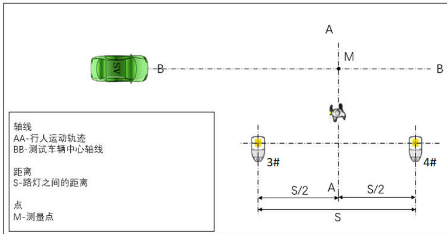
图 B.11 背景照度测量
