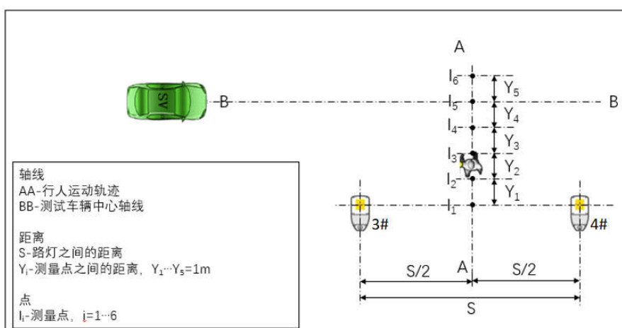
图 B.13 行人路径照度测量
