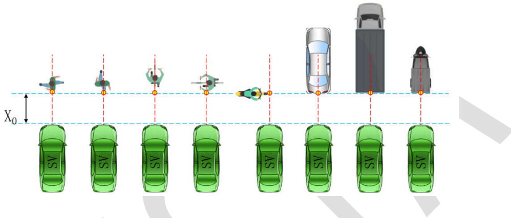
图 2 纵向距离示意图
