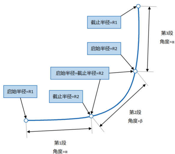
图 A.5 主车左转路径要求
