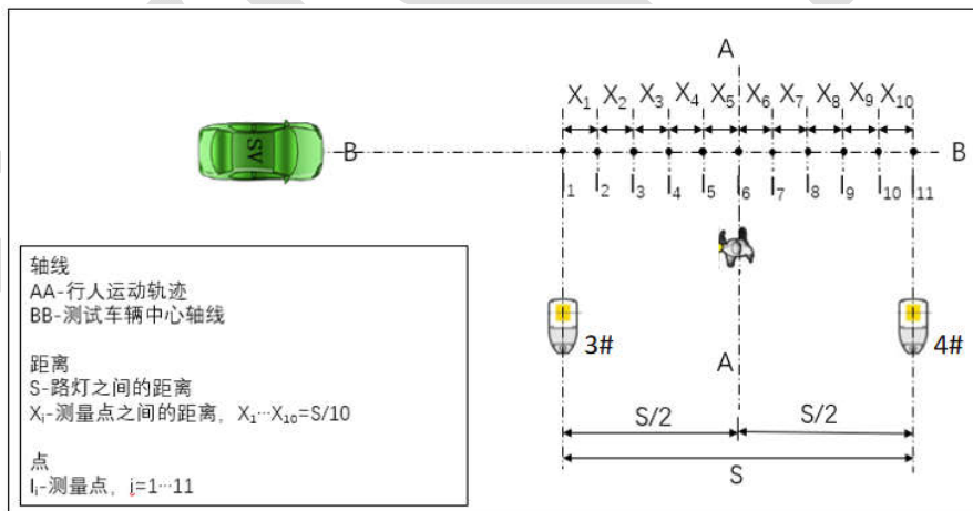
图 B.12 主车路径上的照度测量
