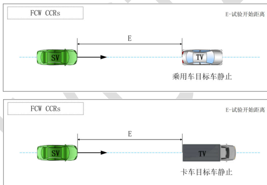
图 A.1 FCW 目标车静止工况
