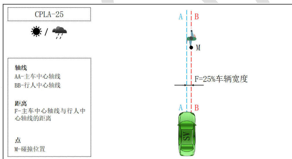
图 B.1 CPLA-25 工况
