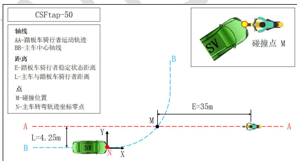
图 B. 9 CSFtap-50 工况
