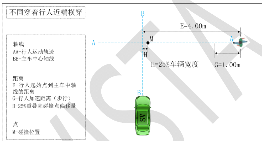
图 C.2 不同穿着行人近端横穿工况
