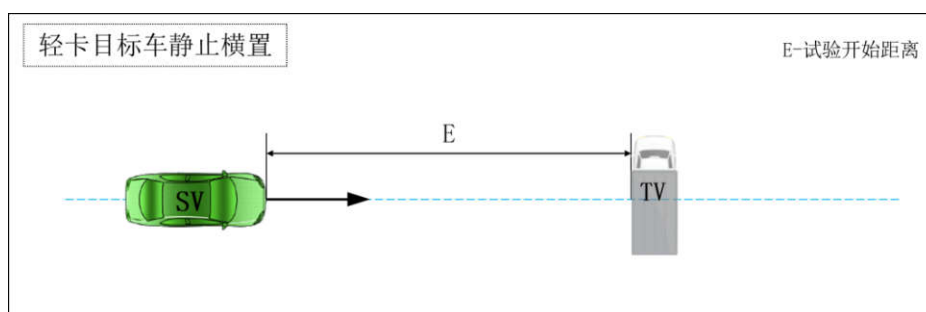
图 C.3 轻卡目标车静止横置工况
