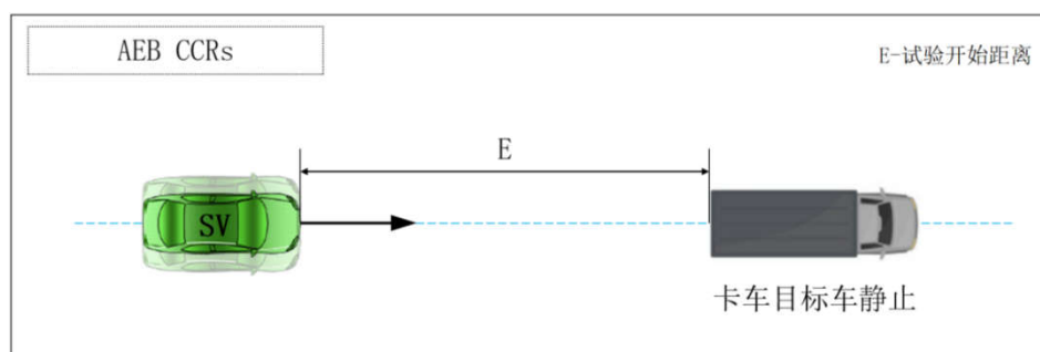
图 A. 6 卡车目标车静止工况
